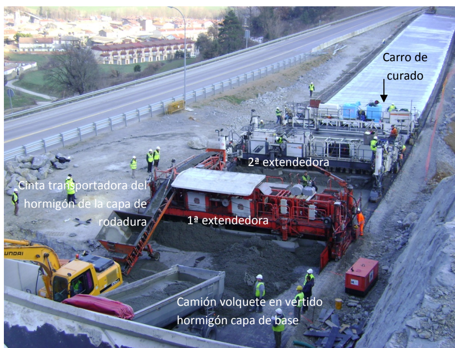
Figura 3.13.- Vista aérea del equipo de extendido y el suministro de los hormigones
