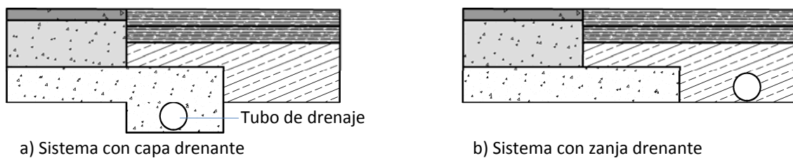
Figura 2.12.- Tipos de arceles
