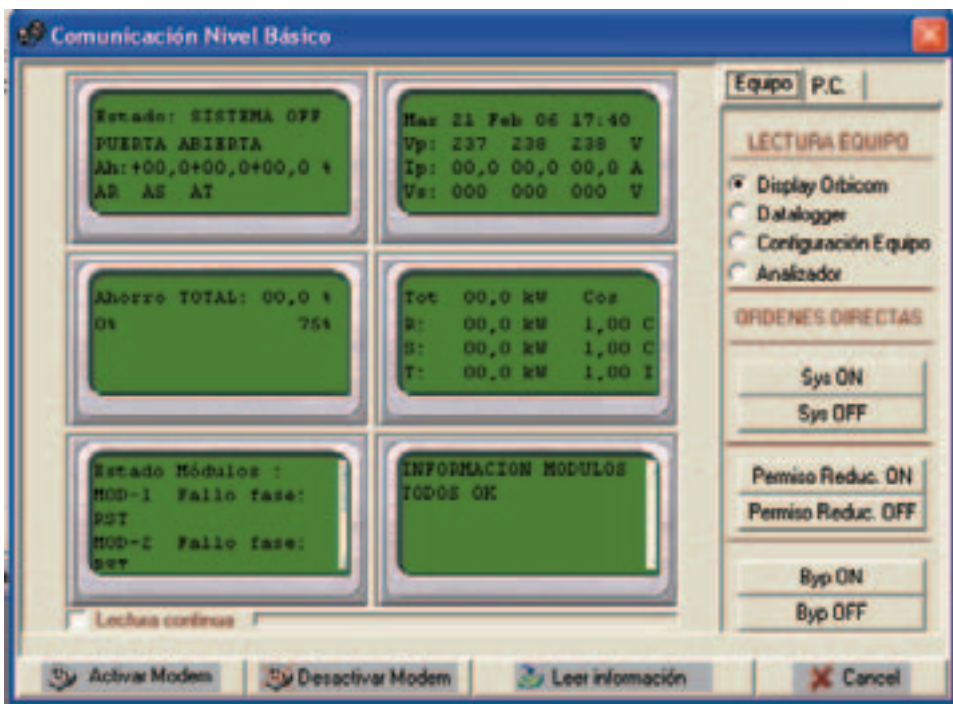
Figura 5. Pantallas de información del sistema de telegestión
