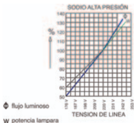
Figura 2. Variación de la potencia y flujo luminosos en función de la tensión en una lámpara VSAP.
