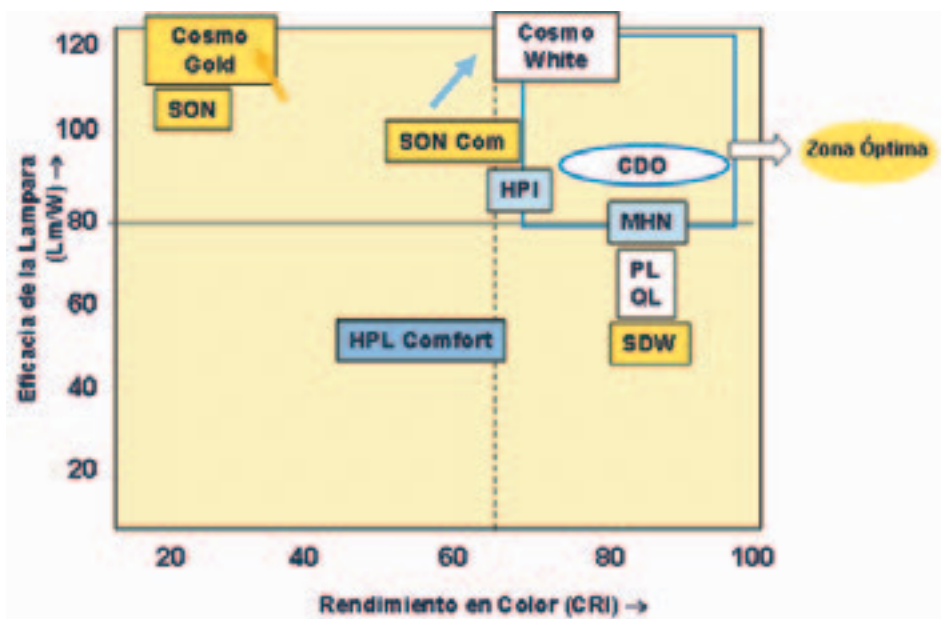
Figura 1. Cuadro comparativo de eficacia de las lámparas.
