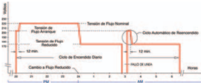
Figura 3. Curva de régimen de arranque, normal y reducido con corte de red en un reductor de flujo.
