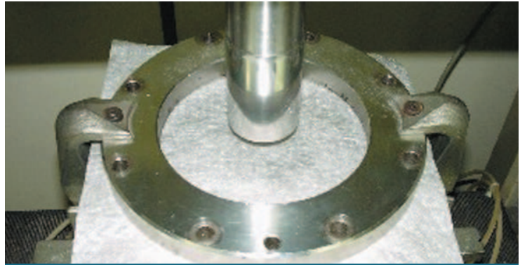
Ensayo de punzonamiento estático (CBR) de un geotextil no tejido.
