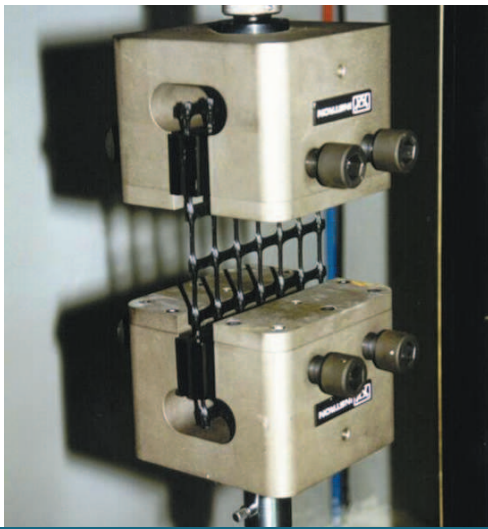
Ensayo de resistencia a tracción de una geomalla.
