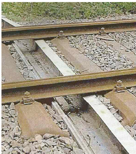
Photos 25 et 26 : A gauche : Une demi-buse posée sous la voie ferrée
