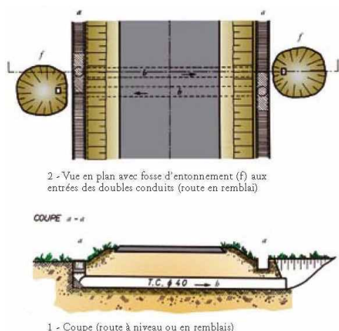
Figure 7 : Schéma de principe d'un passage de type II a. (Source : Guide technique Aménagement et Mesures pour la petite faune, Sétra 2005).
