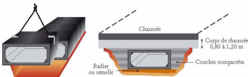
Figure 9 : Schéma d'un passage de type II b avec cadre fermé (Source : Guide technique Aménagements et Mesures pour la petite faune, Sétra 2005)
